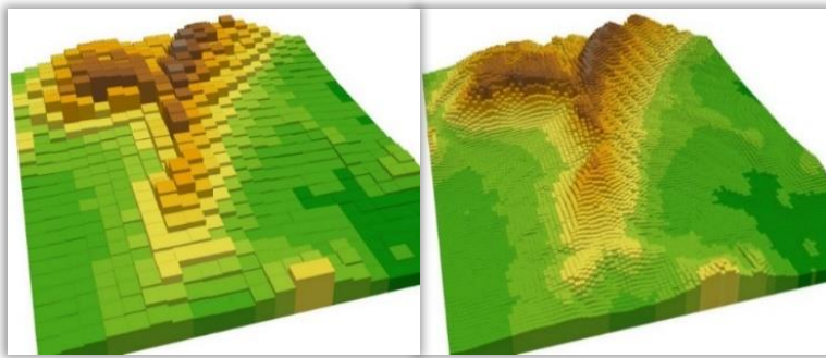
Abbildung 6: Unterschiedliche Rasterweiten (links: 500 m x 500 m; rechts: 125 m x 125 m) bei einem digitalem Geländehöhenmodell
