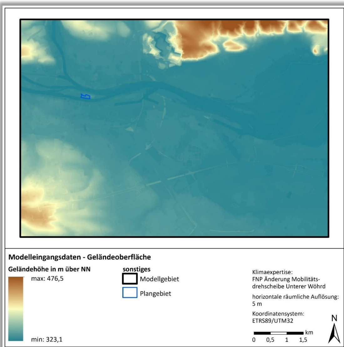
Abbildung 8: Digitales Geländemodell für das Modellgebiet in 5 m-Auflösung.
