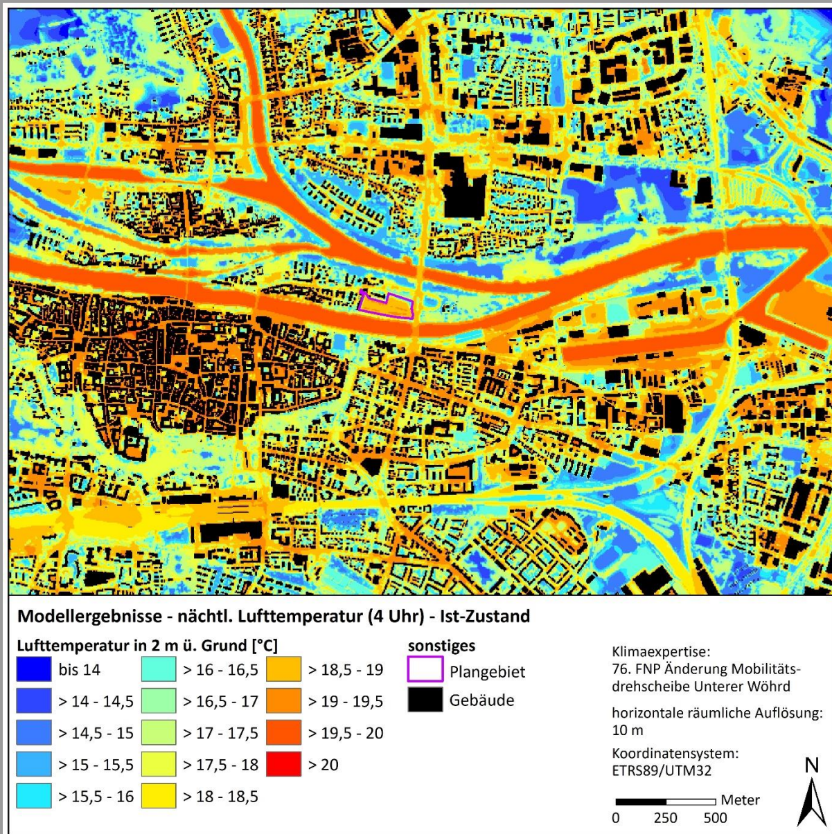
Abbildung 9: Ausprägung der nächtlichen Lufttemperatur im Ist-Zustand.
