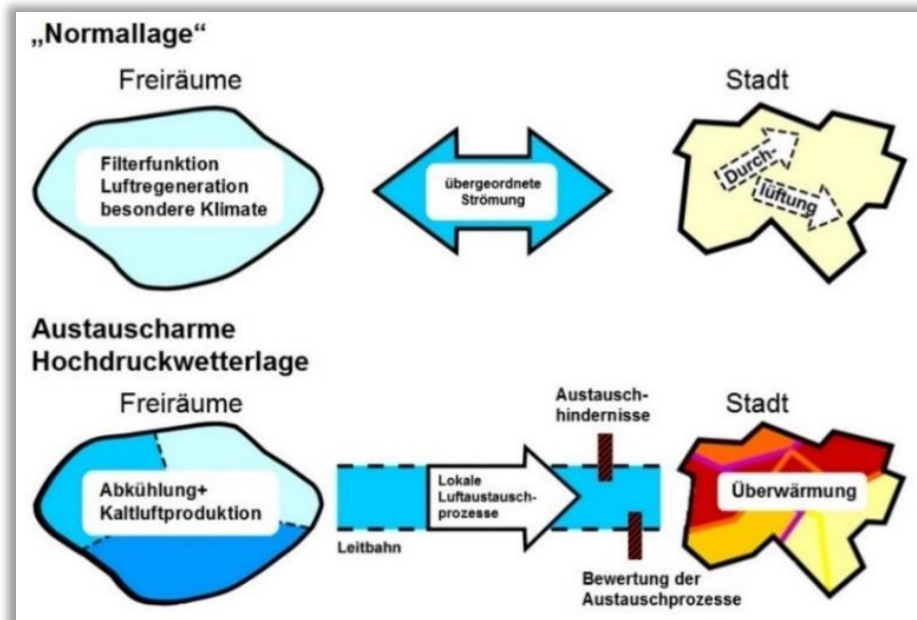
Abbildung 1: Prozessorientierte Analyse bei einer austauscharmen Hochdruckwetterlage
