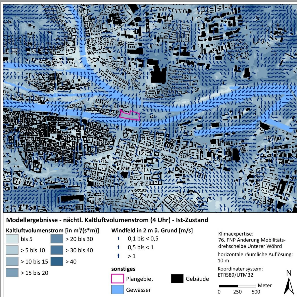
Abbildung 11: Ausprägung des nächtlichen Kaltluftvolumenstroms im Ist-Zustand.
