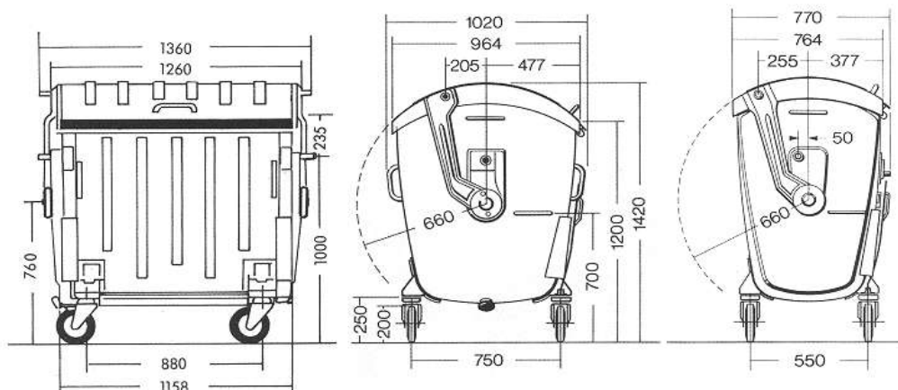
770- und 1100l-MGB
