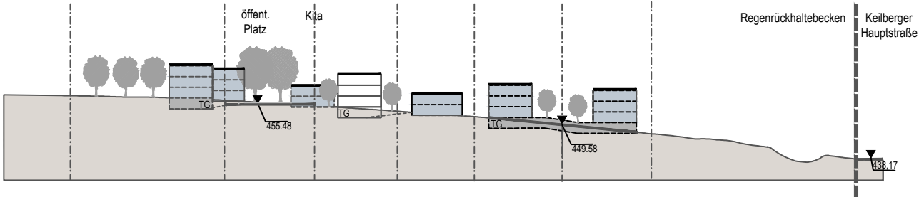
Schnitt A-A (Schematisch)
