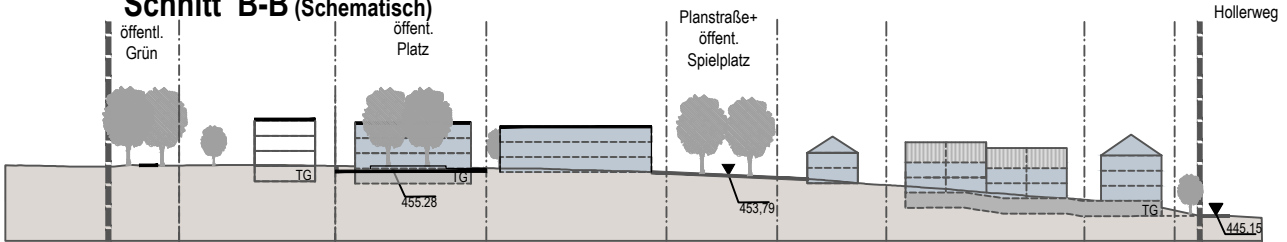
Schnitt B-B (Schematisch)
