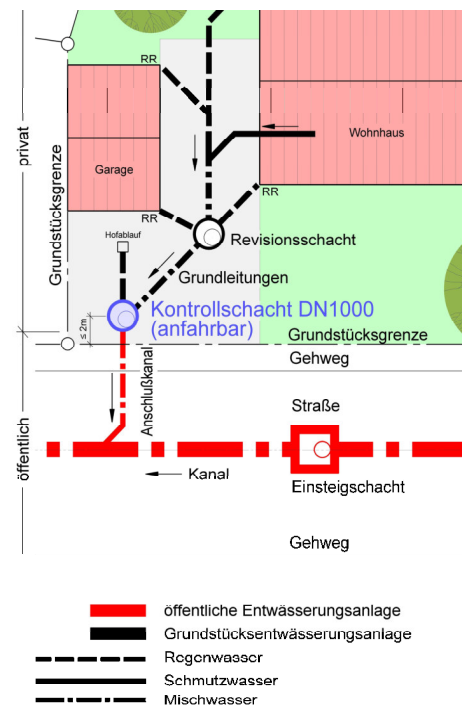
Beispiel Grundstücksentwässerungsanlage
