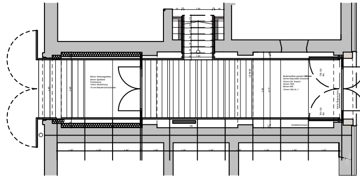
Grundriss Passage
