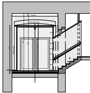
Schnitt Zugang Poststelle
